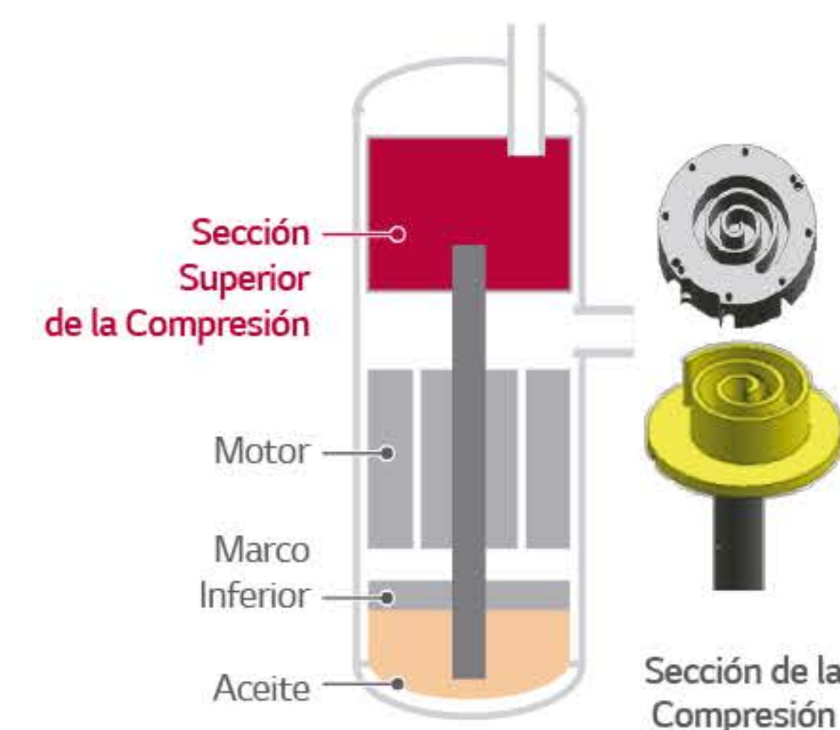
COMPRESOR SCROLL CONVENCIONAL
