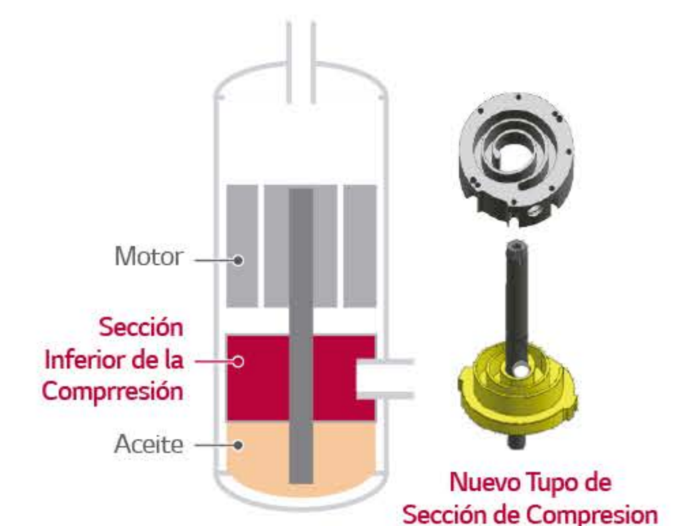
COMPRESOR R1™
